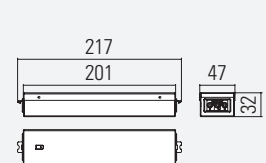
JUNCTION BOX (DISPLAY 3000/F6)
