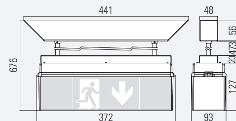
L01P PENDELMONTAGE
