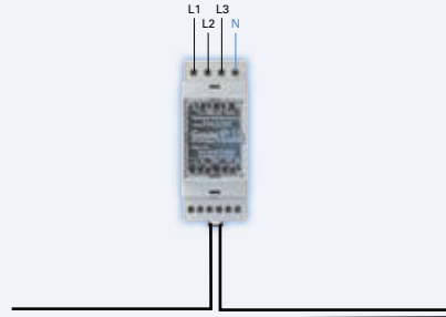
Überwachung des AV-Netzes (3 phasig)
