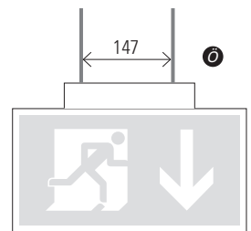
Ösenmontage
