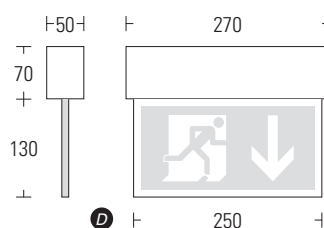
Ösenmontage
