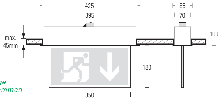
Deckeneinbau
